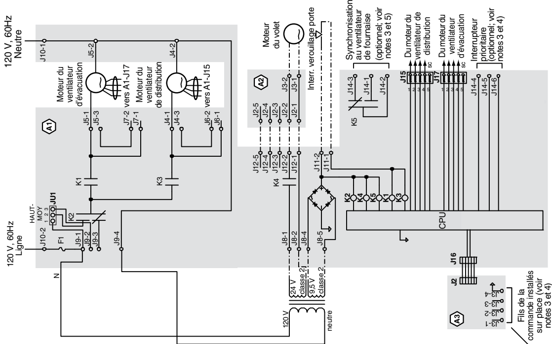
SCHÉMA LOGIQUE
