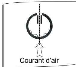
Alignement du distributeur de vapeur dans un conduit vertical pour le SKR-30/40
